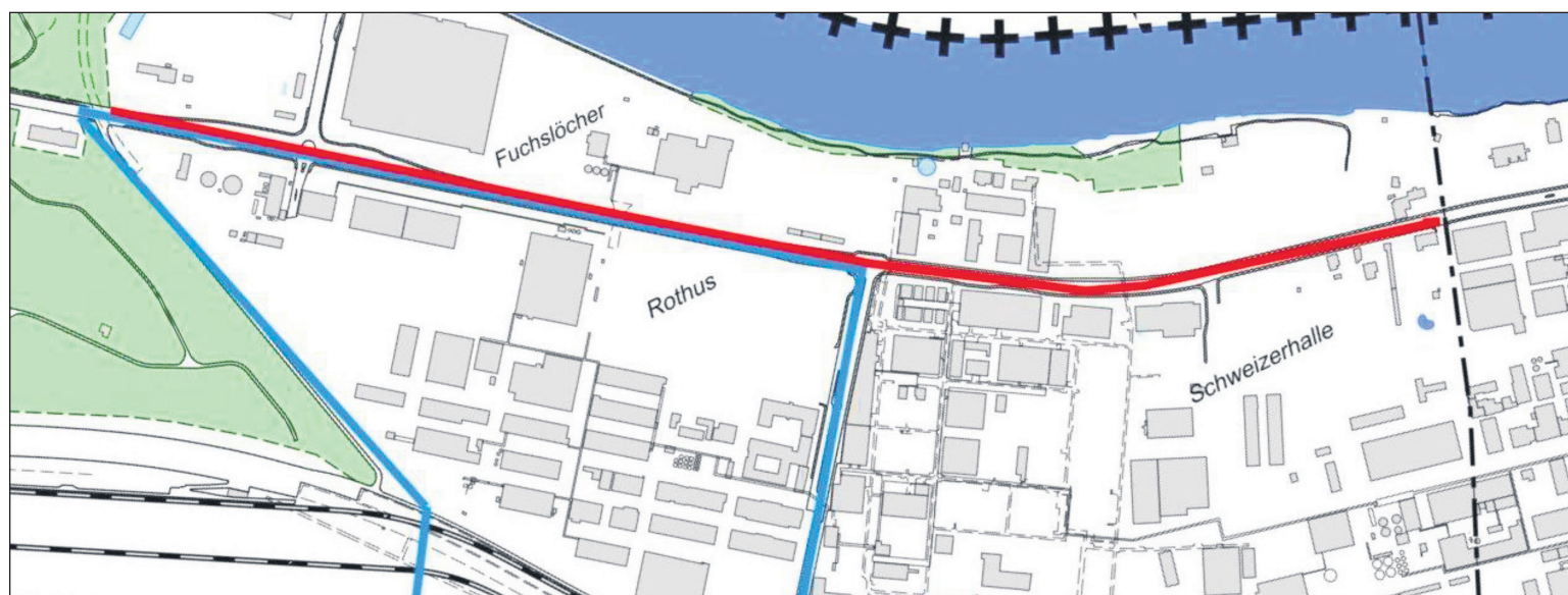
Abb. 1 Perimeter Sanierung Rheinfelderstrasse und schematische Darstellung Transportwasserleitungen, Ausschnitt Geoportall
