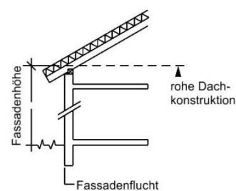
a) Detail Messweise Fassadenhöhe
