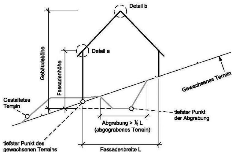
b) Detail Messweise Gebäudehöhe
