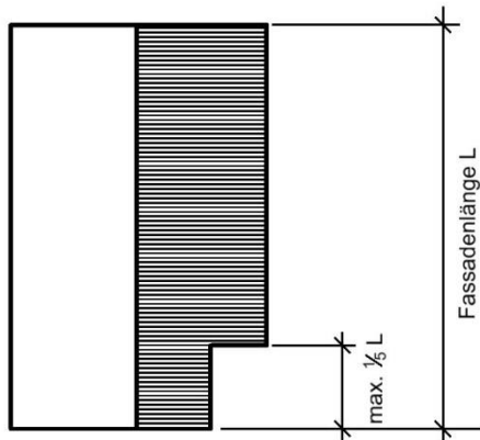
a) Aufsicht
